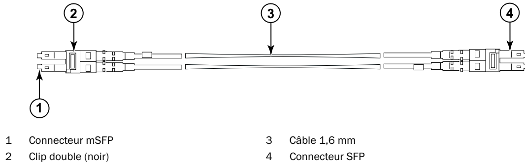
FIGURE 6 Conception de câble pour les câbles de raccordement mSFP pour la lame FC8-64 à port haute densité
